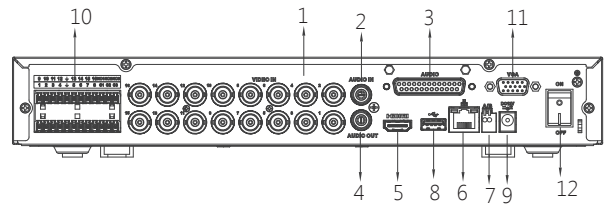
DH-XVR7116HE-4KL-X
