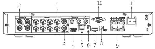
DH-XVR7108HE-4KL-X
